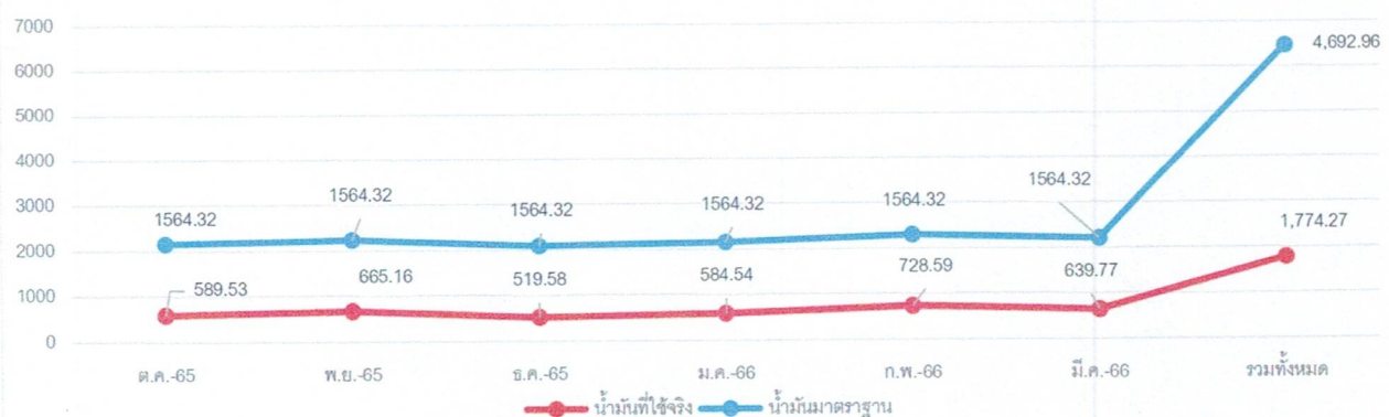
กราฟแสดงการใช้พลังงานเชื้อเพลิง ปีงบประมาณ พ.ศ.2566 (ต.ค.65 - มี.ค.66)
